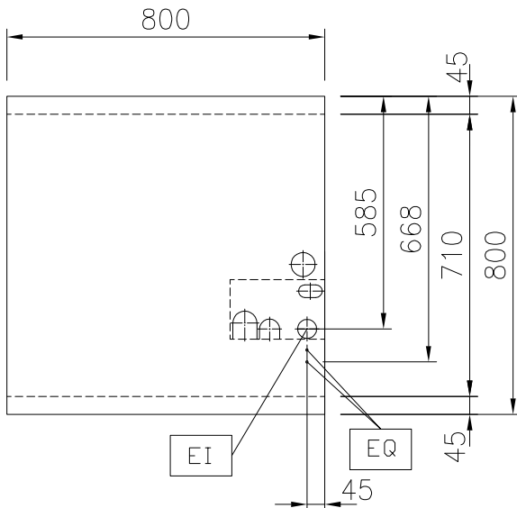
Boven aanzicht
