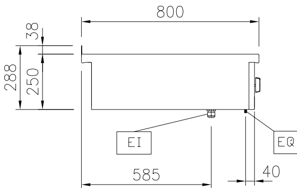
Zij aanzicht
